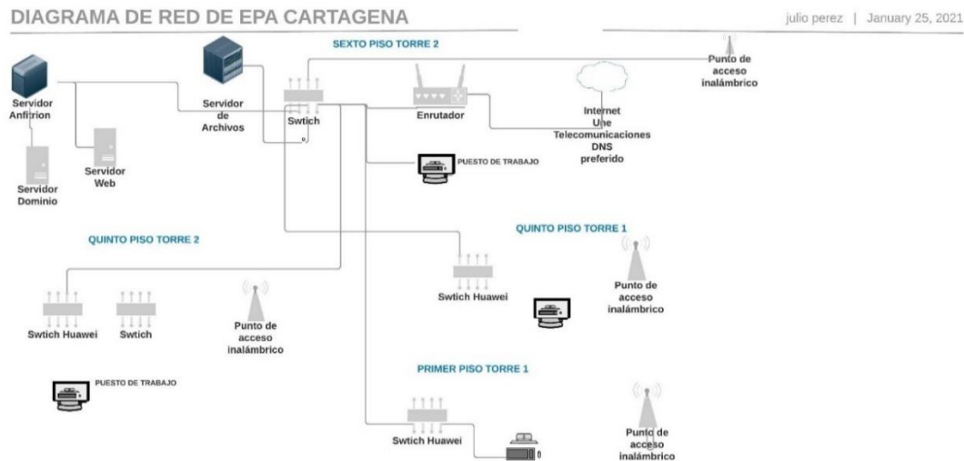
Grafica 3. Diagrama de red de EPA Cartagena.
