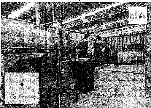
Tanque preparación del aditivo y tanque de almacenamiento
